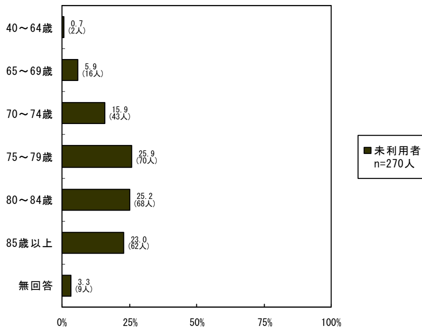
図7.3 年齢
