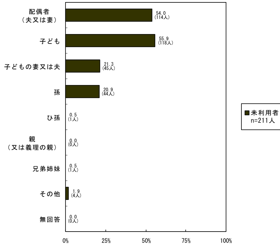
図7.8.3 同居家族
