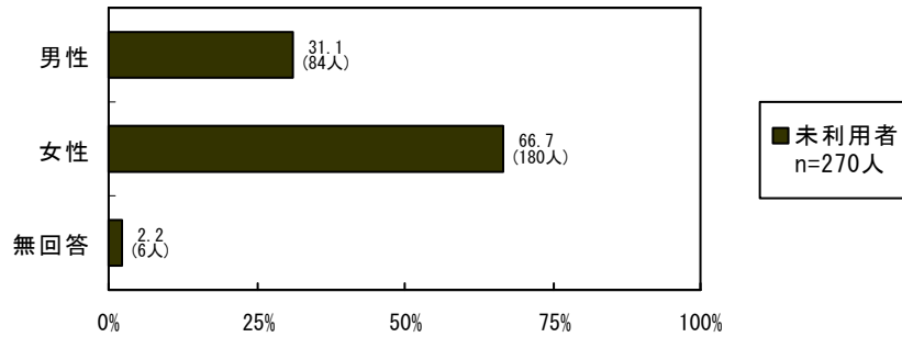
図7.2 性別
