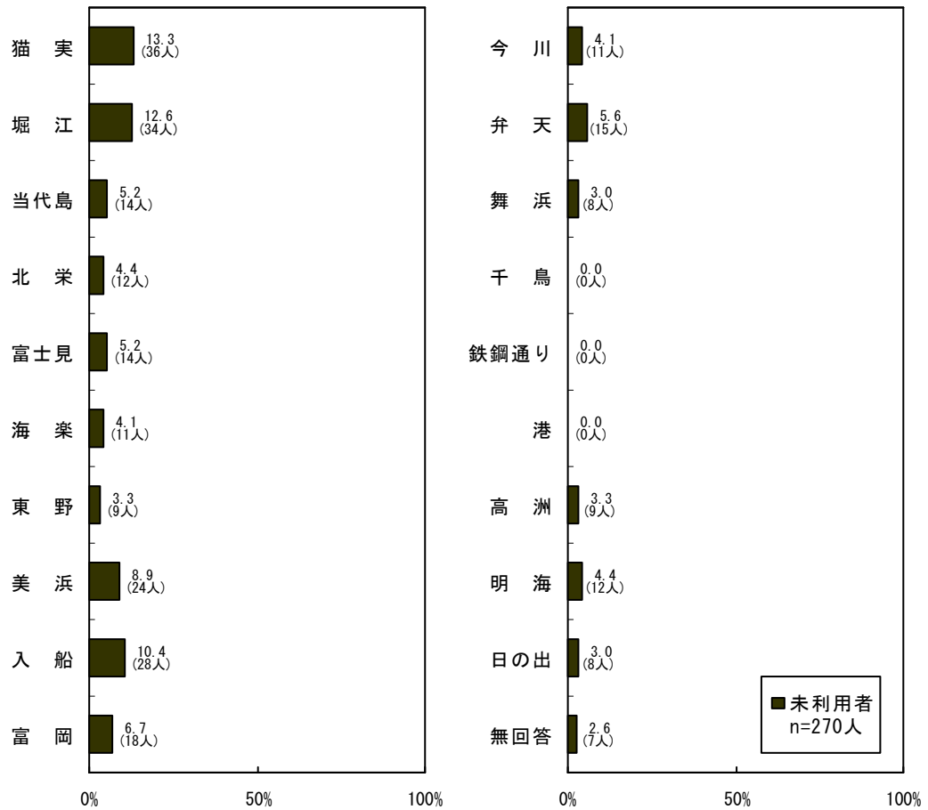
図7.7 居住地区
