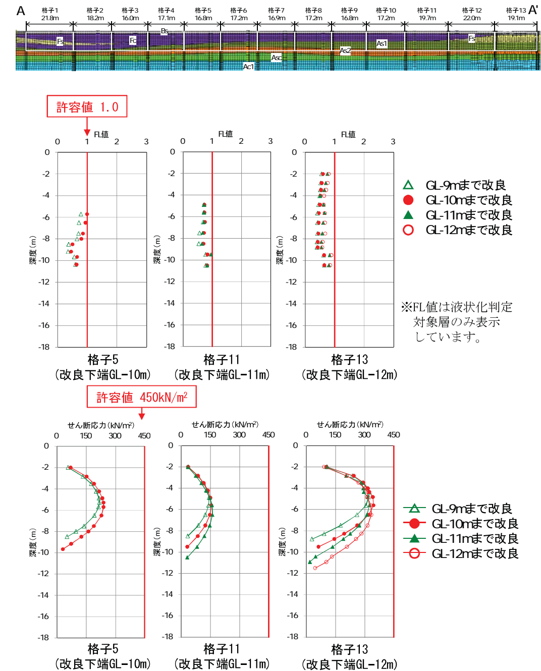
図-2.11 FL値と改良体に発生するせん断応力最大値の深度分布 (レベル2地震動 A-A'断面)
