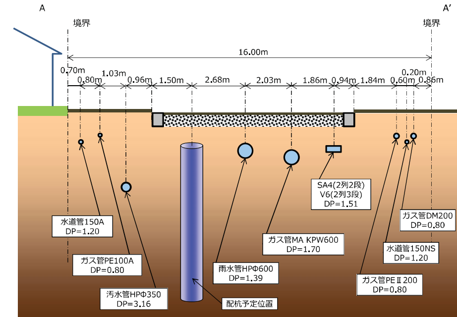
図-2.3(1) 道路内断面図(A-A'断面)
