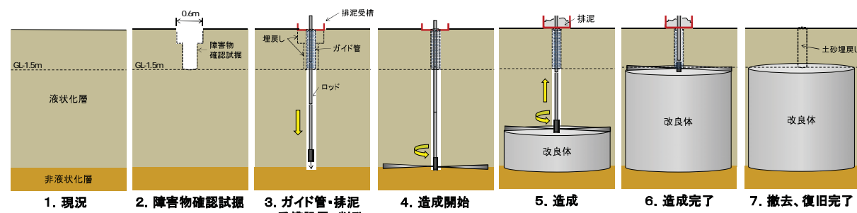
図-2.13 高圧噴射攪拌工法の施工手順 (宅地部を標準)
