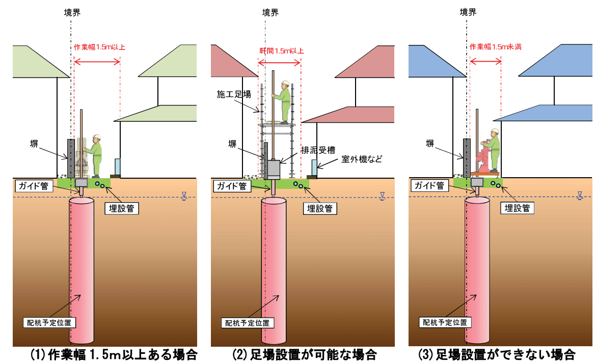
図-2.4 宅地内の改良体配置断面イメージ図
