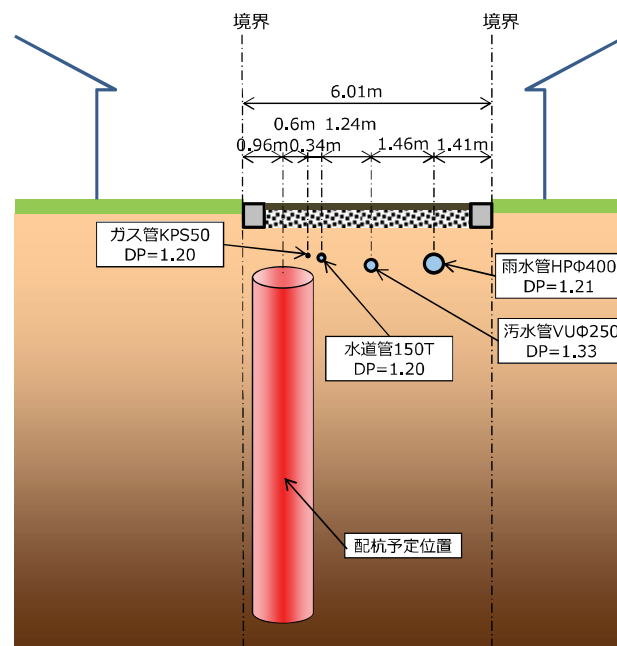
図-2.3(4) 道路内断面図 (D-D' 断面)
