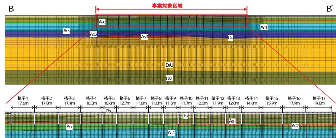
図-2.5(2) B-B' 断面の擬似3次元解析モデル (上: 全体、下: 対策範囲拡大)
