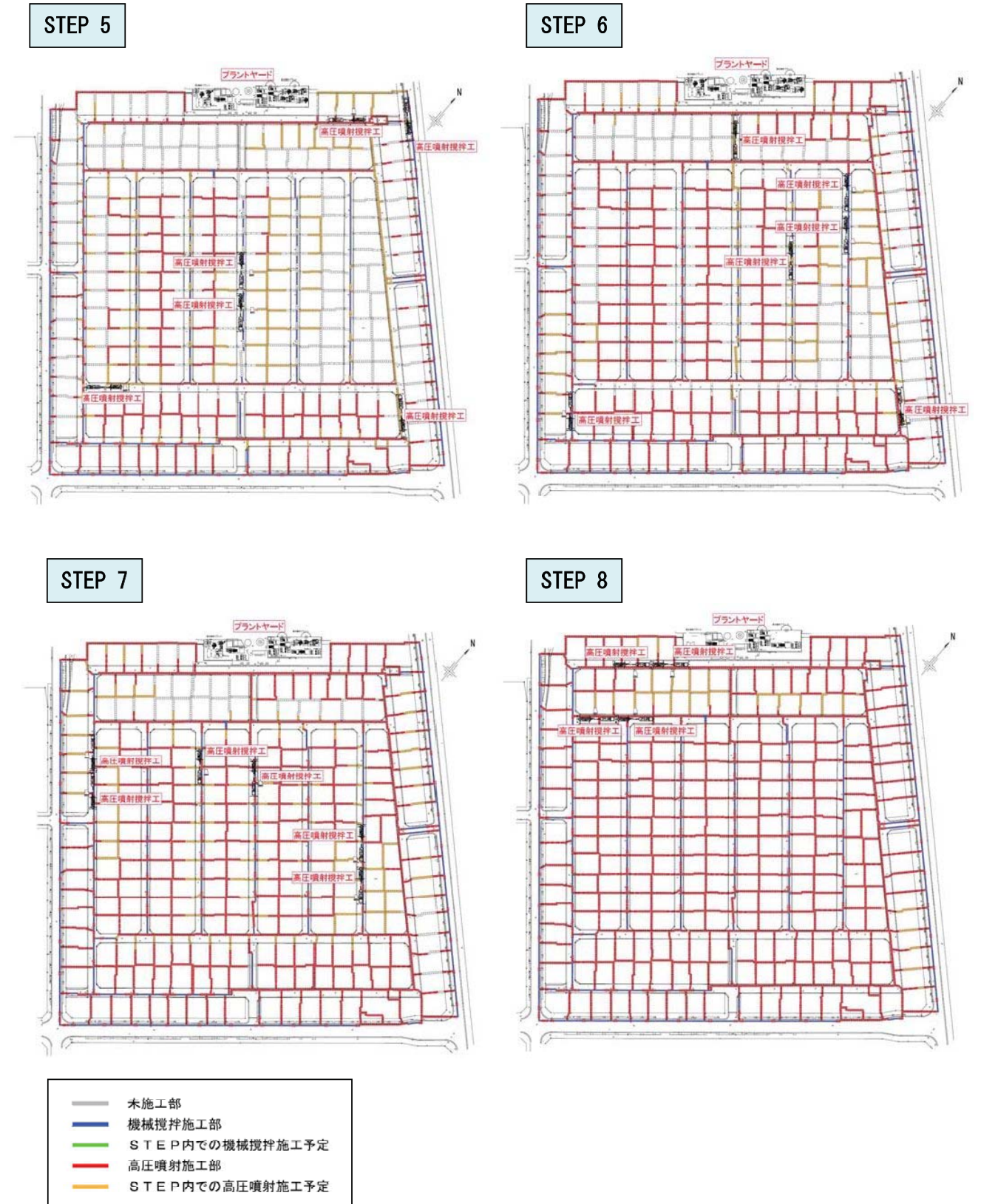
図-2.18(2) 各STEPにおける施工状況と機械配置例
