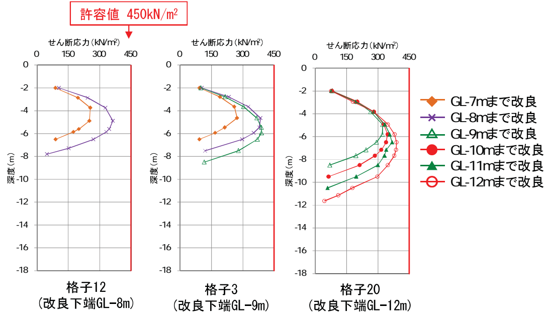
図-2.11(1) FL値と改良体が発生するせん断応力最大値の深度分布 (レベル2地震動 A-A'断面)
