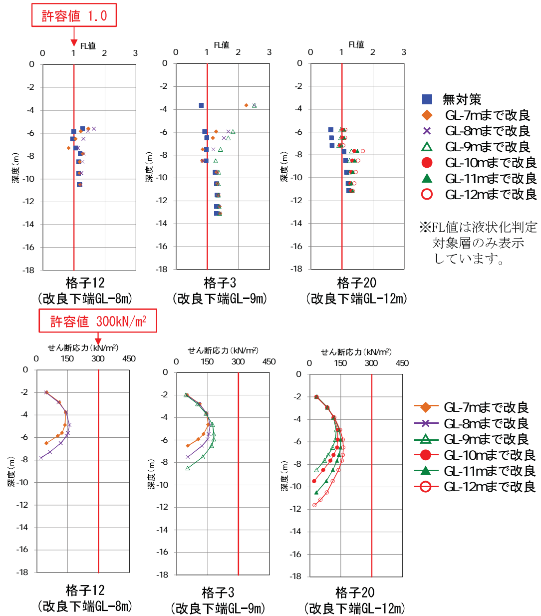
図-2.10(1) FL値と改良体に発生するせん断応力最大値の深度分布 (対策対象地震動 A-A'断面)
