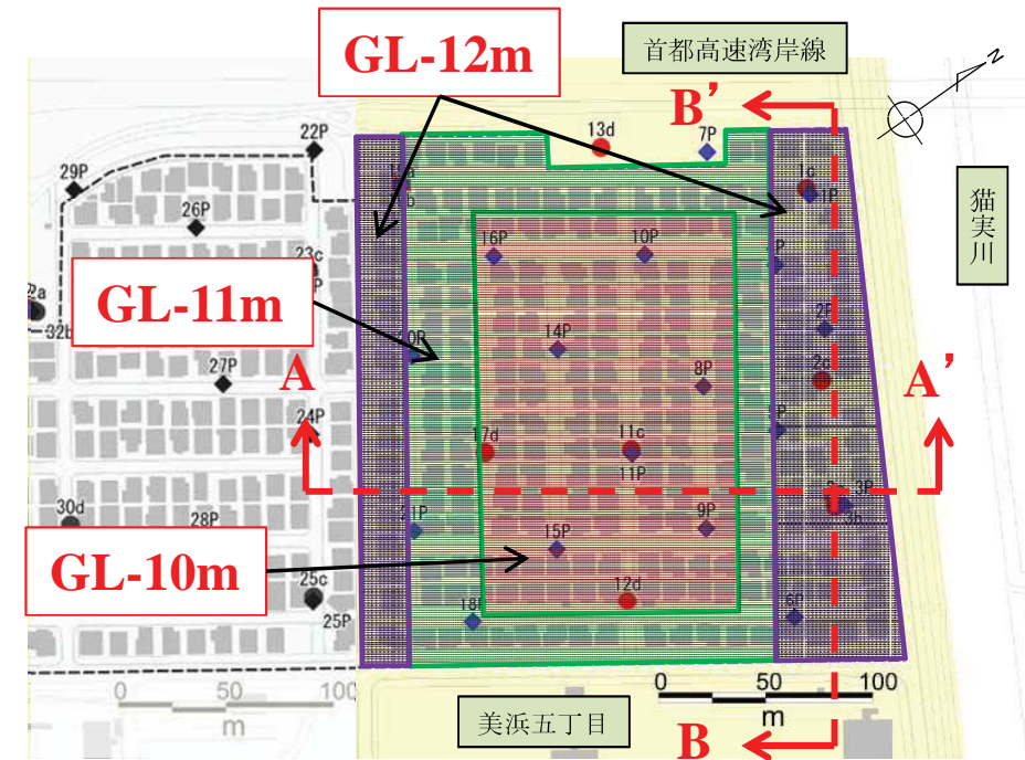
図-2.9 改良体下端深度の平面分布図
