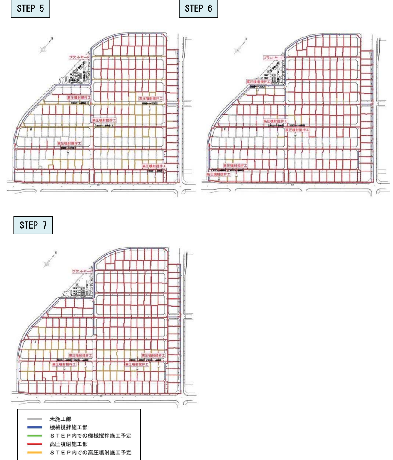
図-2.18(2) 各STEPにおける施工状況と機械配置例
