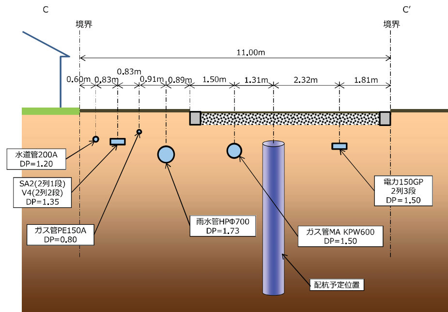
図-2.3(3) 道路内断面図 (C-C' 断面)
