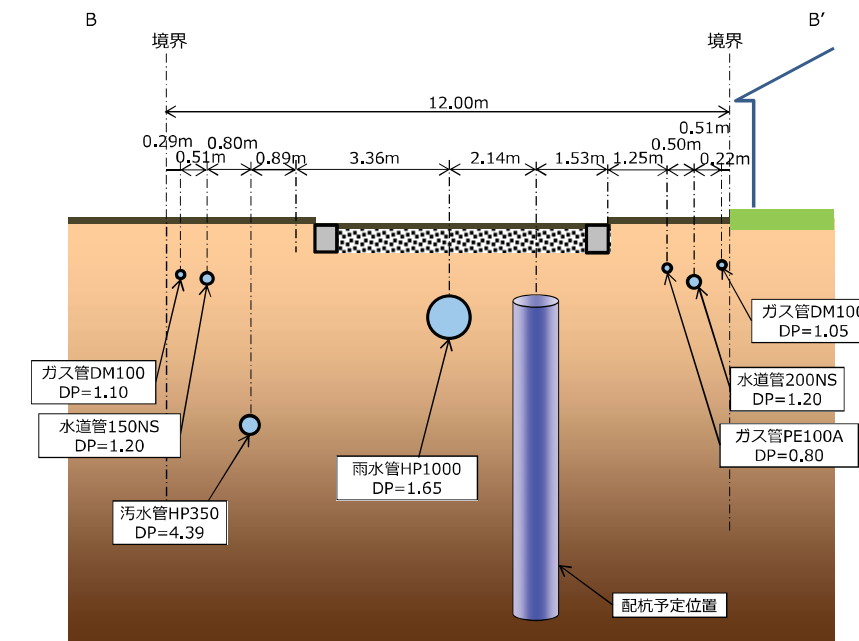
図-2.3(2) 道路内断面図(B-B'断面)
