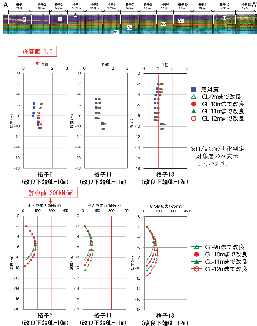
図-2.10 FL値と改良体に発生するせん断応力最大値の深度分布 (対策対象地震動 A-A'断面)
