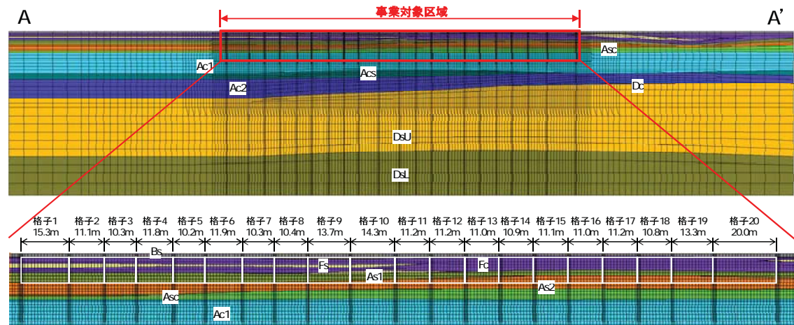
図-2.5(1) A-A' 断面の擬似3次元解析モデル (上: 全体、下: 対策範囲拡大)
