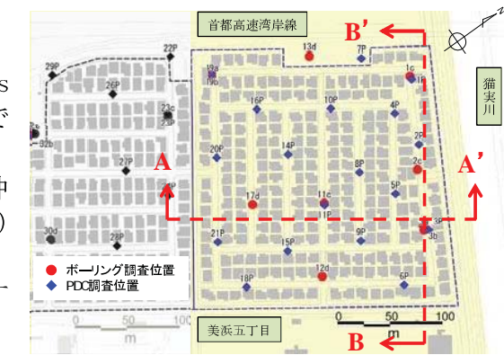
図-1.4 地盤断面位置図
