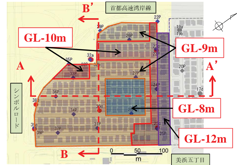
図-2.9 改良体下端深度の平面分布図
