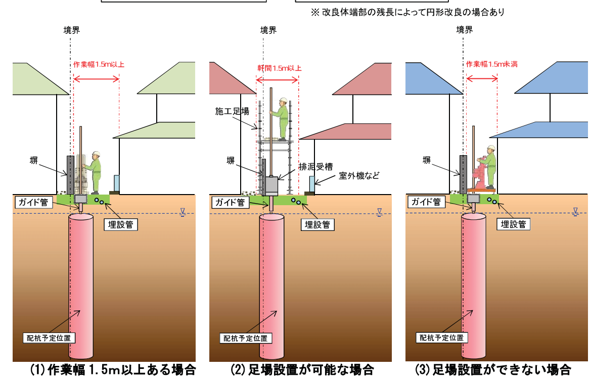
図-2.4 宅地内の改良体配置断面イメージ図
