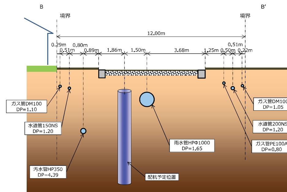
図-2.3(2) 道路内断面図(B-B'断面)
