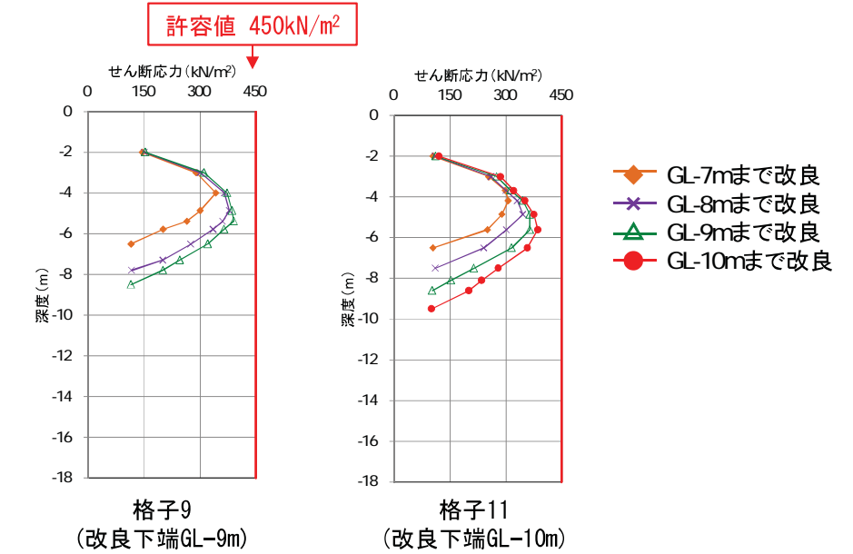
図-2.11(2) FL値と改良体が発生するせん断応力最大値の深度分布 (レベル2地震動 B-B'断面)
