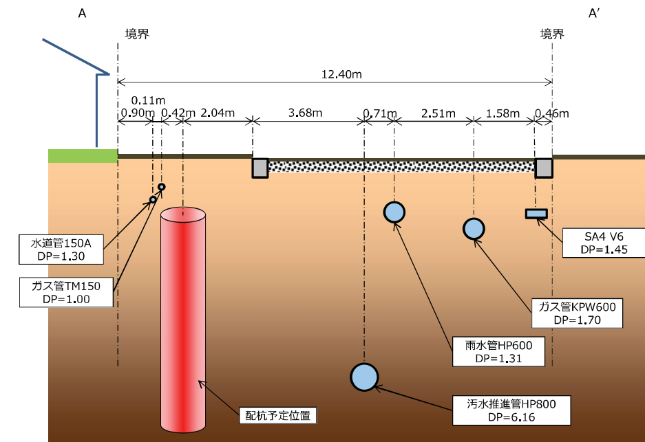
図-2.3(1) 道路内断面図(A-A'断面)
