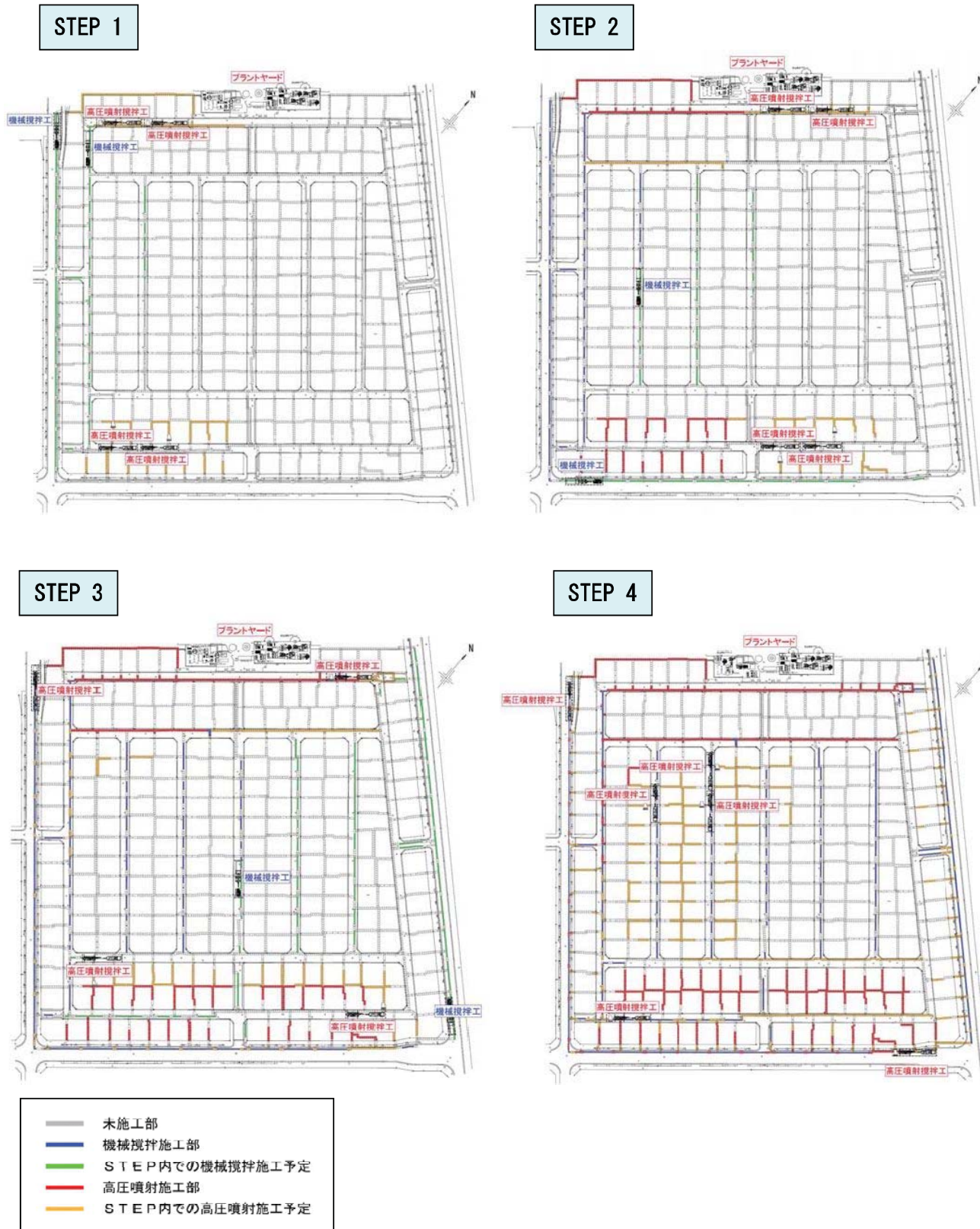
図-2.18(1) 各STEPにおける施工状況と機械配置例
