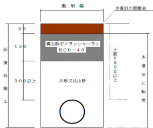
仮復旧構造
