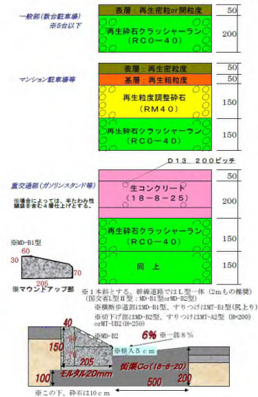
歩道切下げ等に伴う舗装復旧断面図 ※箇所の構造で施工
