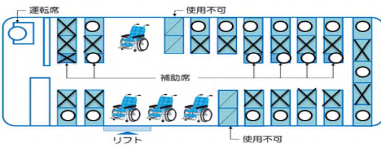
車いす4台 車内レイアウト
