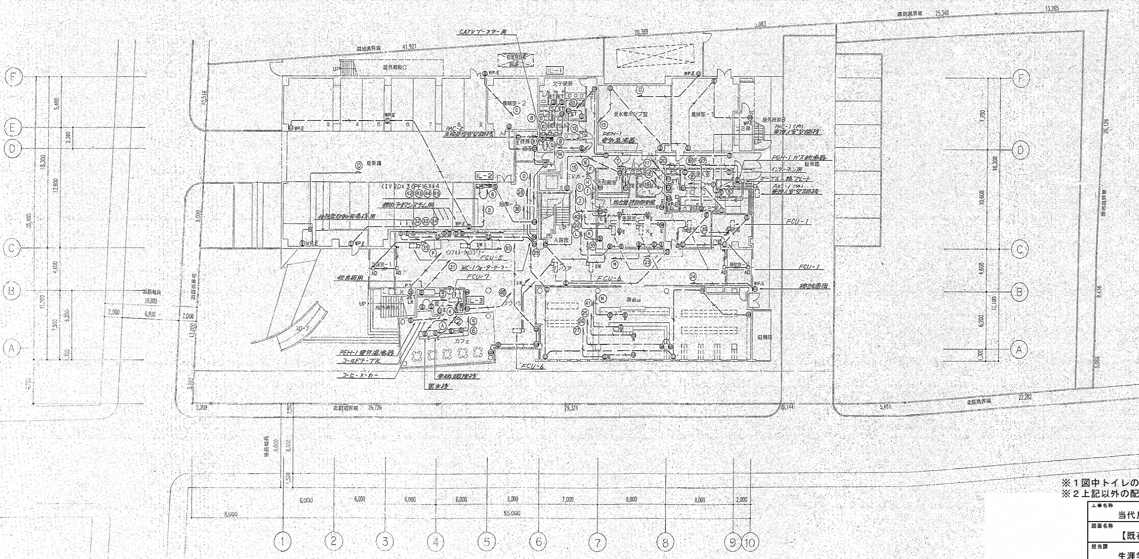
配置 1階平面図 1:200
