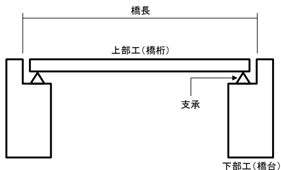
付図－１ 橋梁の基本構成
