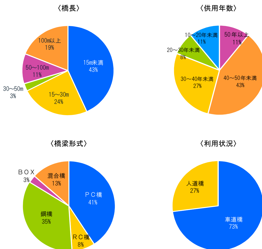
図－3.2 橋梁の分類
