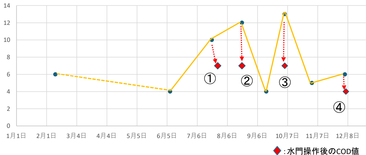
あけぼの橋（水面）COD経年変化と施設操作効果
