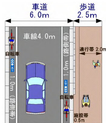
計画道路幅員 8.5m（一般部）
