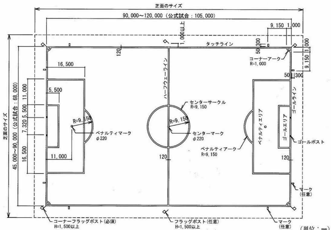
図 6-2-2 サッカー場寸法図
