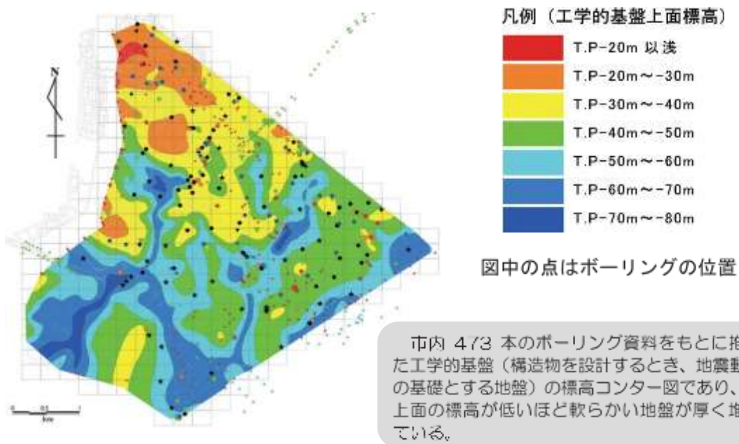
■工学的基盤標高コンター図（平成 23 年度浦安市液状化対策技術検討調査）
